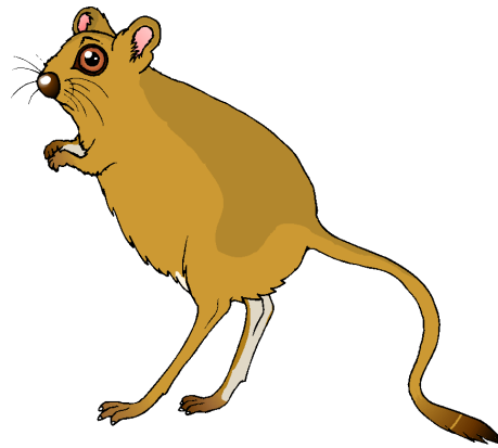
gerbil gerbil
